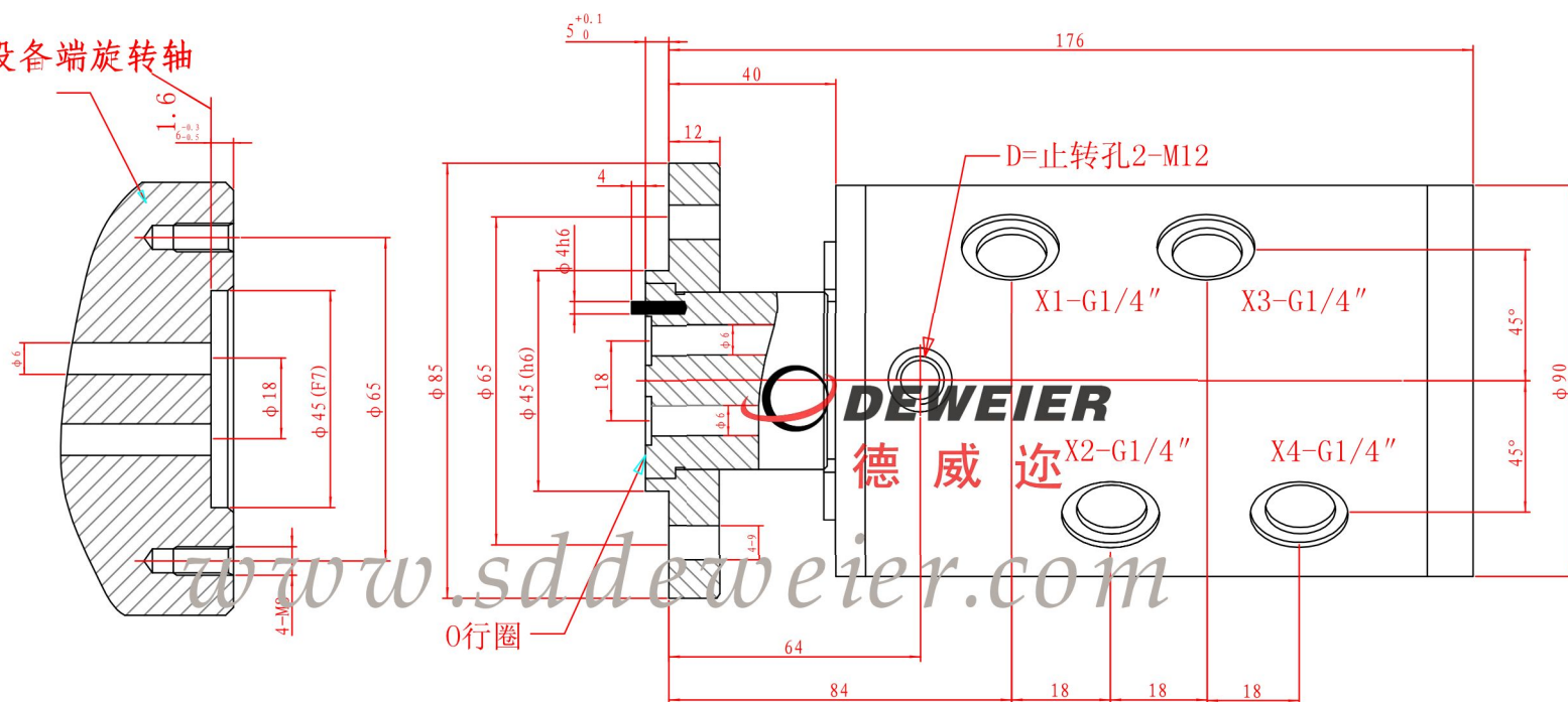
液压四通道旋转接头-DRF04008
